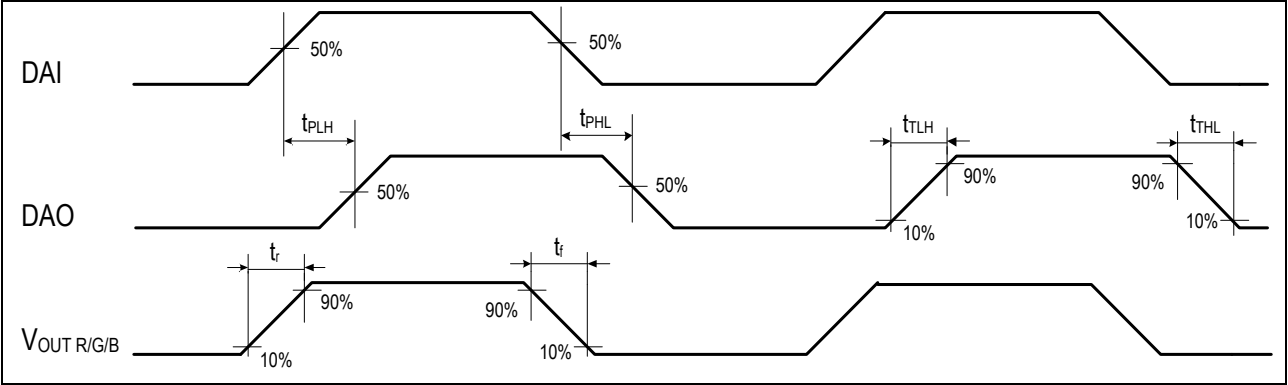
Fig. DMX512AW-B 动态参数测试示意图
