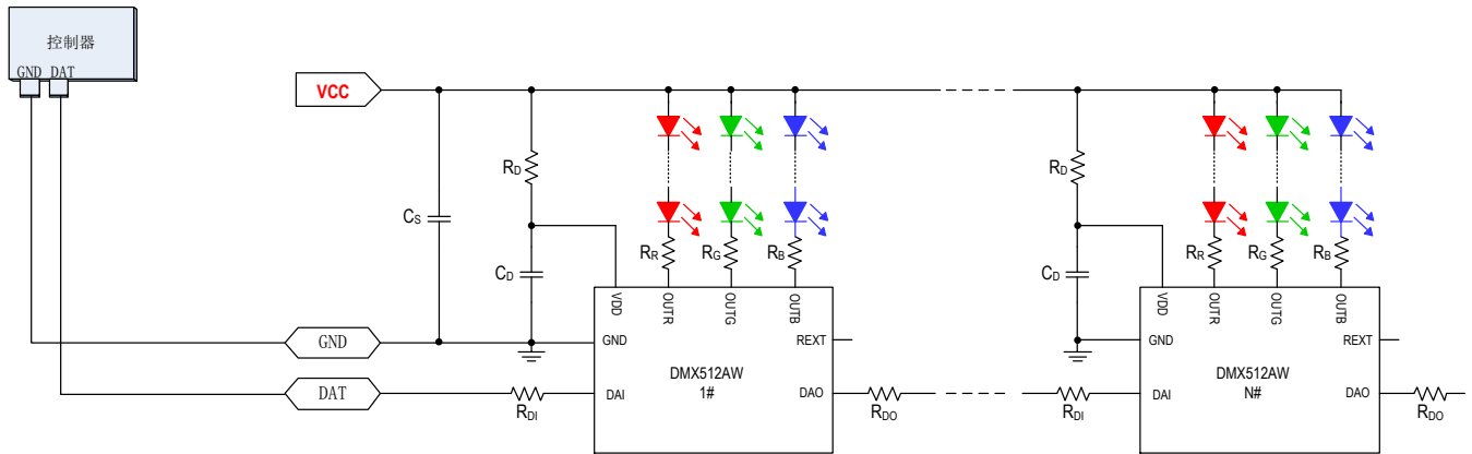
Fig. DMX512AW-B 典型应用方案图
