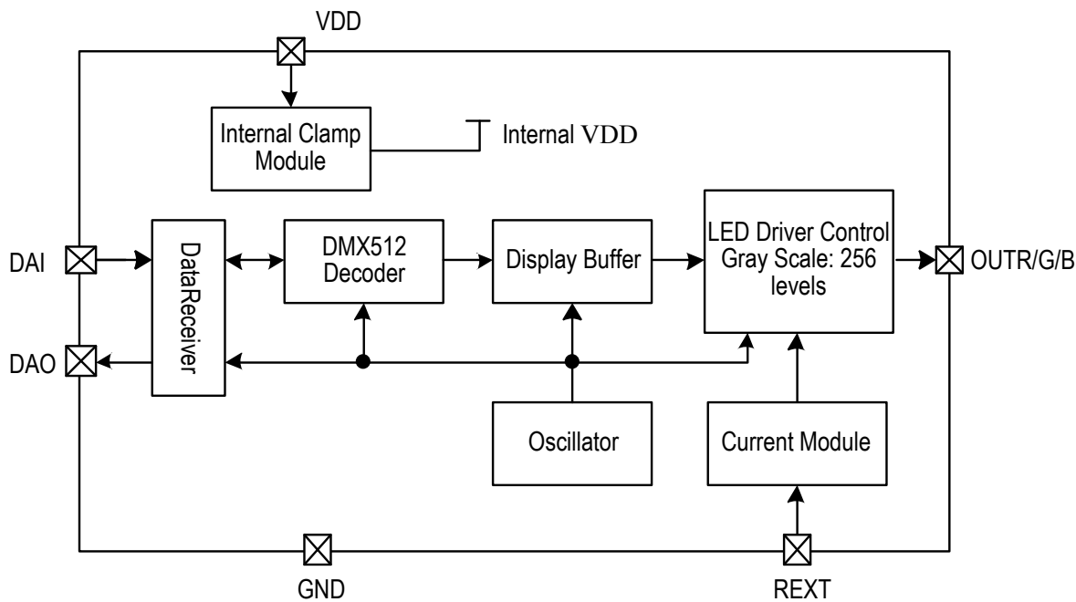
Fig. DMX512AW-B 内部功能框图
