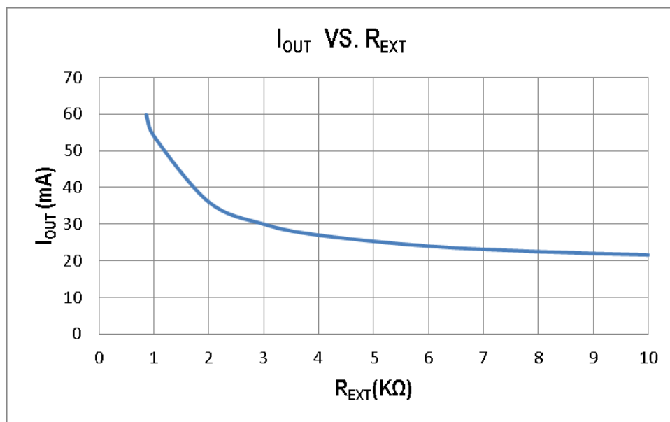
Fig. DMX512AW-B 输出电流 I_{OUT} 与 R_{EXT} 的关系图
