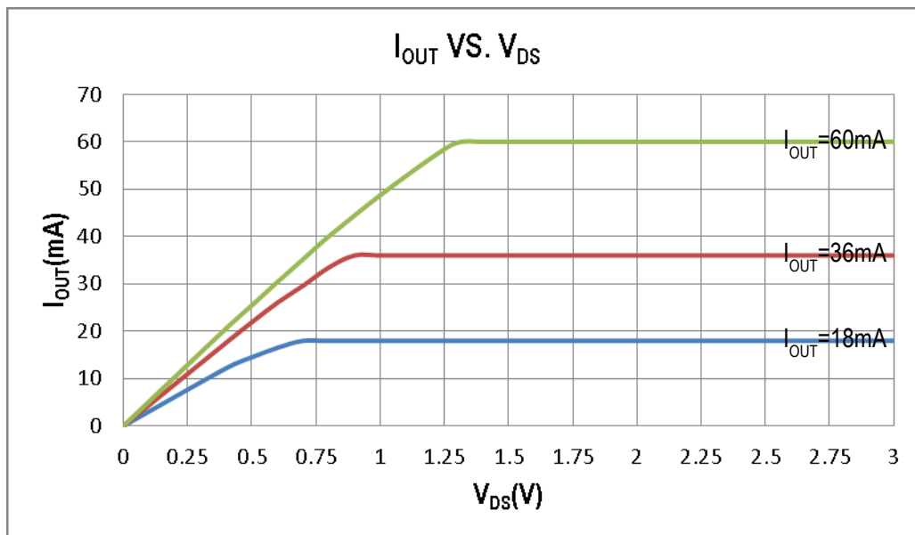
Fig. DMX512AW-B I_{OUT} 与 OUT 端口电压 V_{DS} 的关系图
