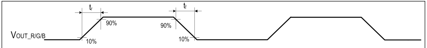
Fig. SM18511PB 动态参数测试示意图
