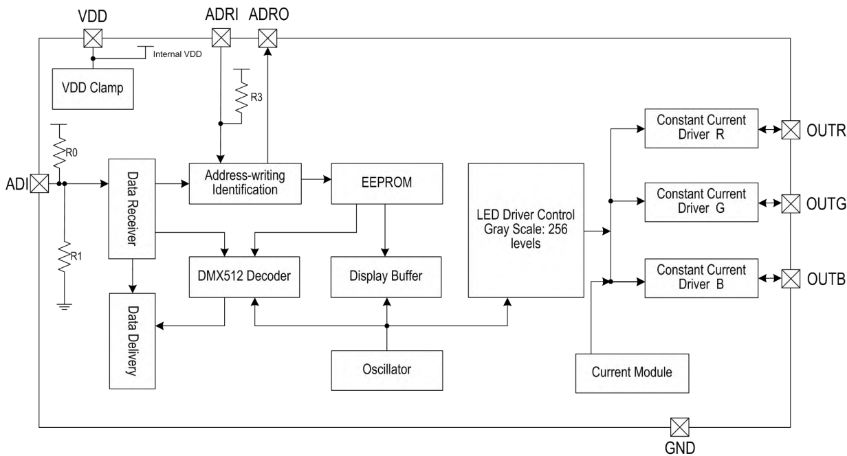
Fig.SM18511PB 内部功能框图
