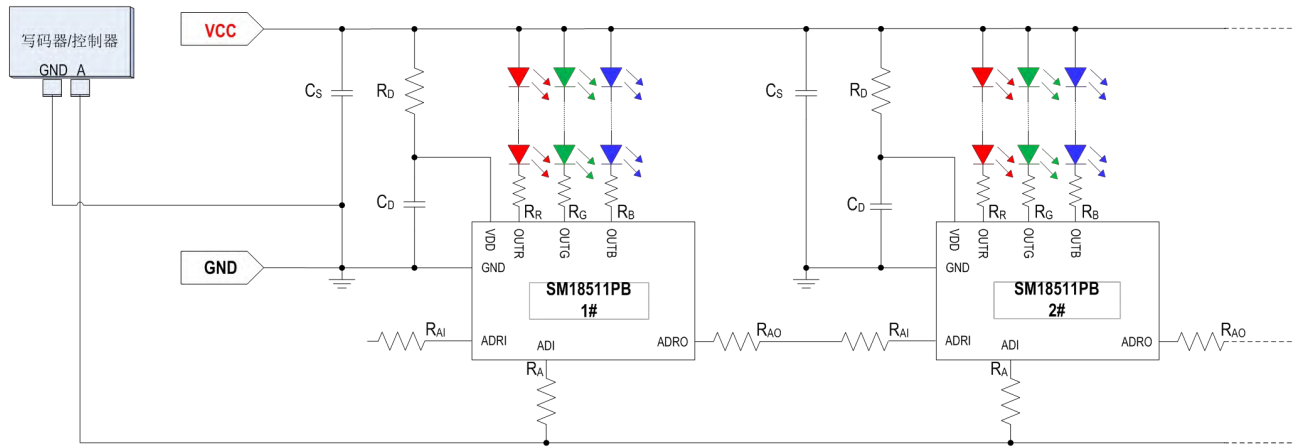
Fig. SM18511PB 典型应用方案图
